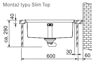
Montaż typu Slim Top
